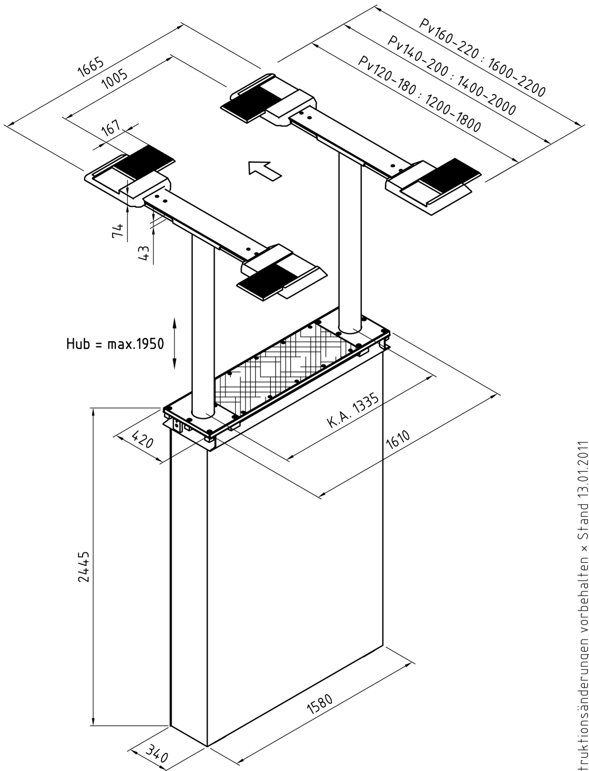
Maßskizze incl. Angabe der Überfahrhöhen
