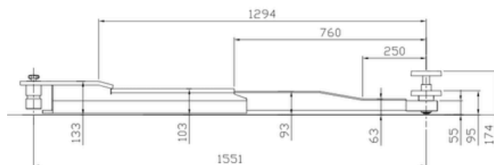
Long arm
